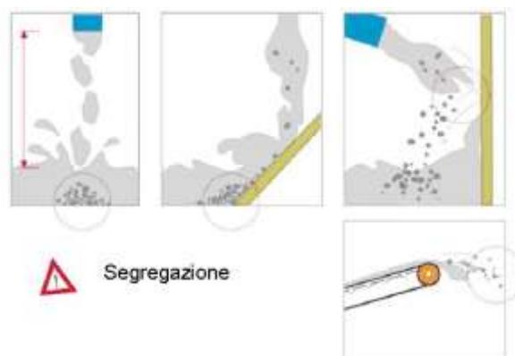
Figura 7: Errori nella posa in opera del calcestruzzo.
